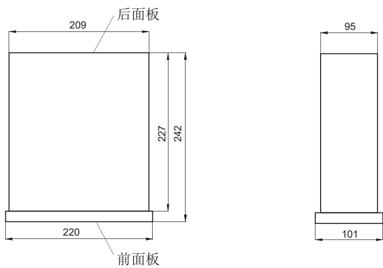
外形尺寸图
