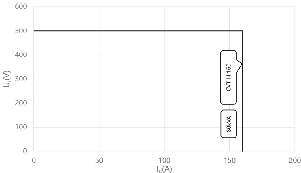
图 4-1 额定级容量与级电压和负载电流的关系
