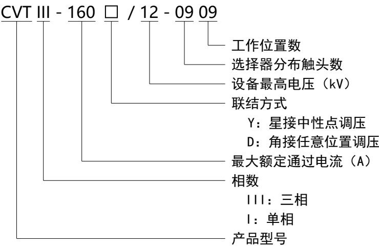
图 3-1 分接开关型号说明
