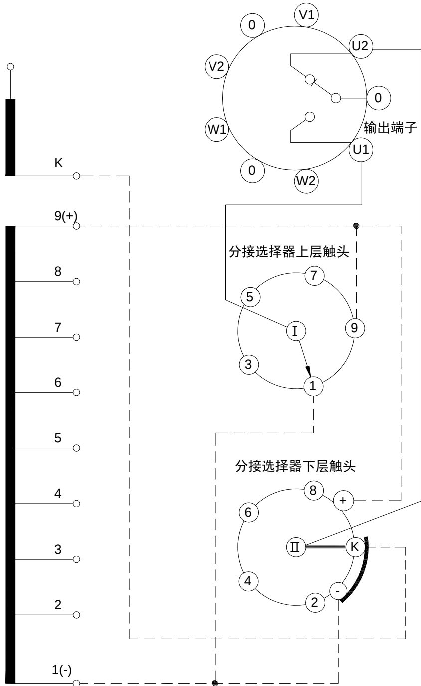
附图 10 VCME 型分接开关±8 级（10193W）工作位置表和接线图
