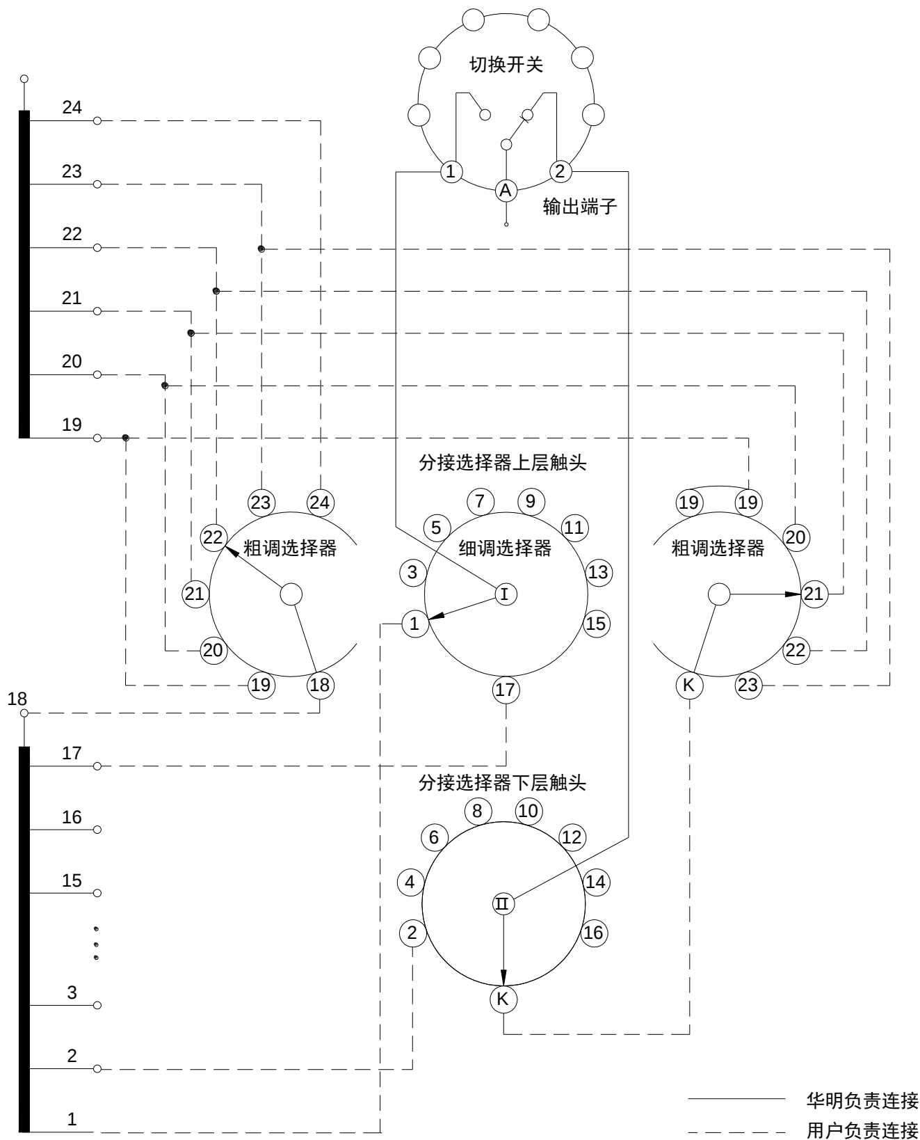
附图 11 VCME 型分接开关 (181071G) 接线图
