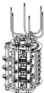
分接选择器
