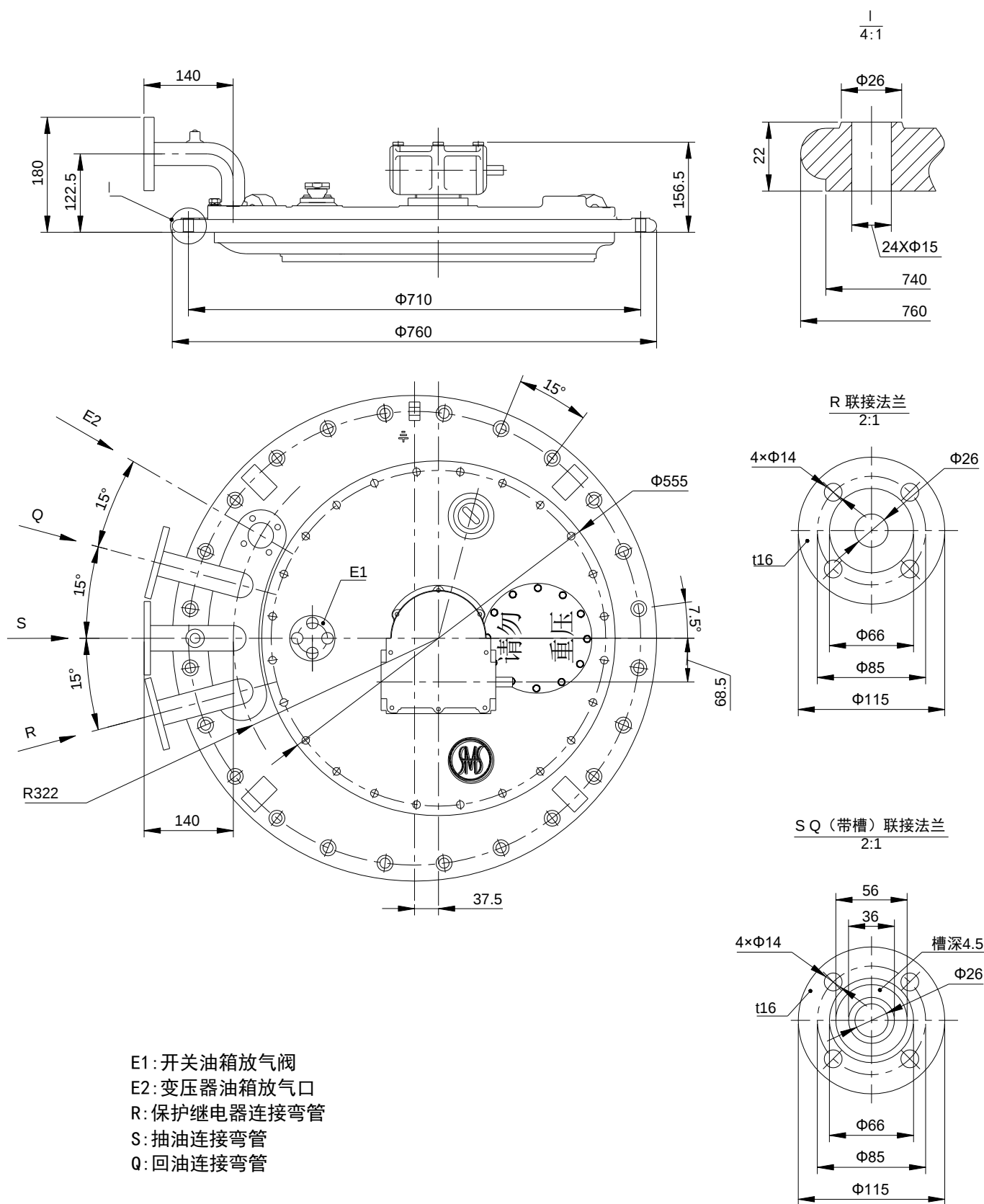
附图 1 VCME 型分接开关安装法兰外形尺寸图
